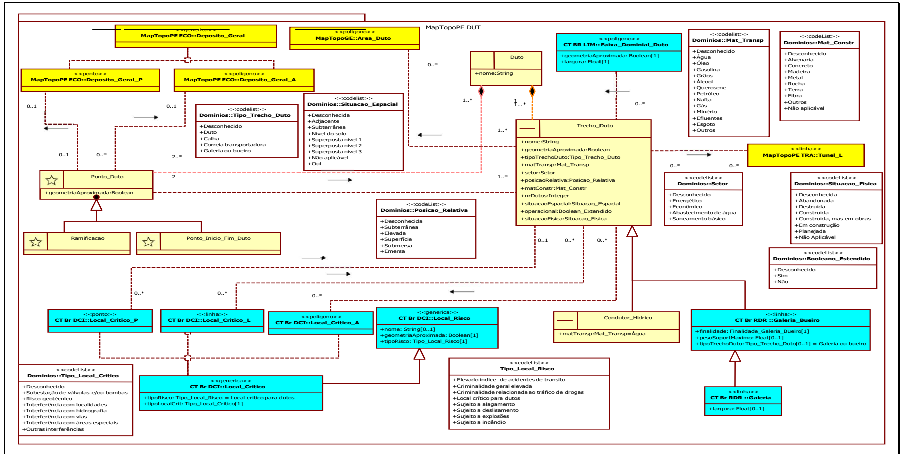
Figura 15. Diagrama de classes para Sistema de Transporte / Dutos.
