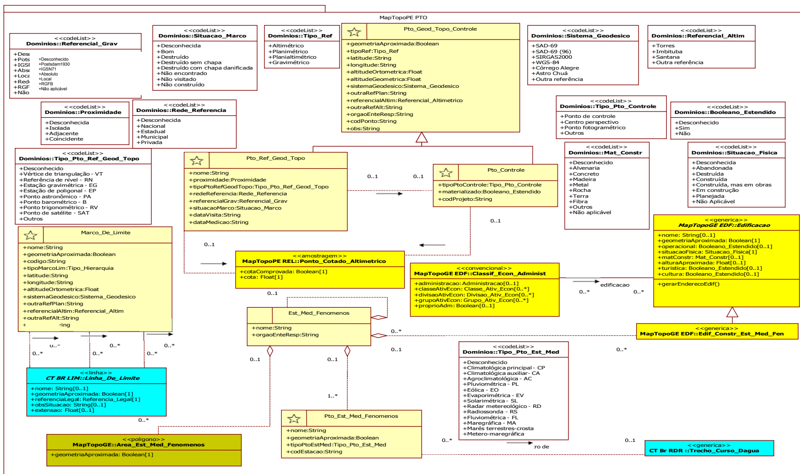
Figura 8. Diagrama de classes para Pontos de Referência.
