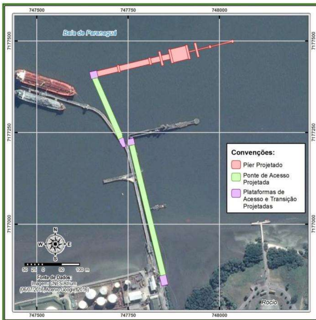
Figura 3.5 – Layout do Pier L - Graneis Líquidos
